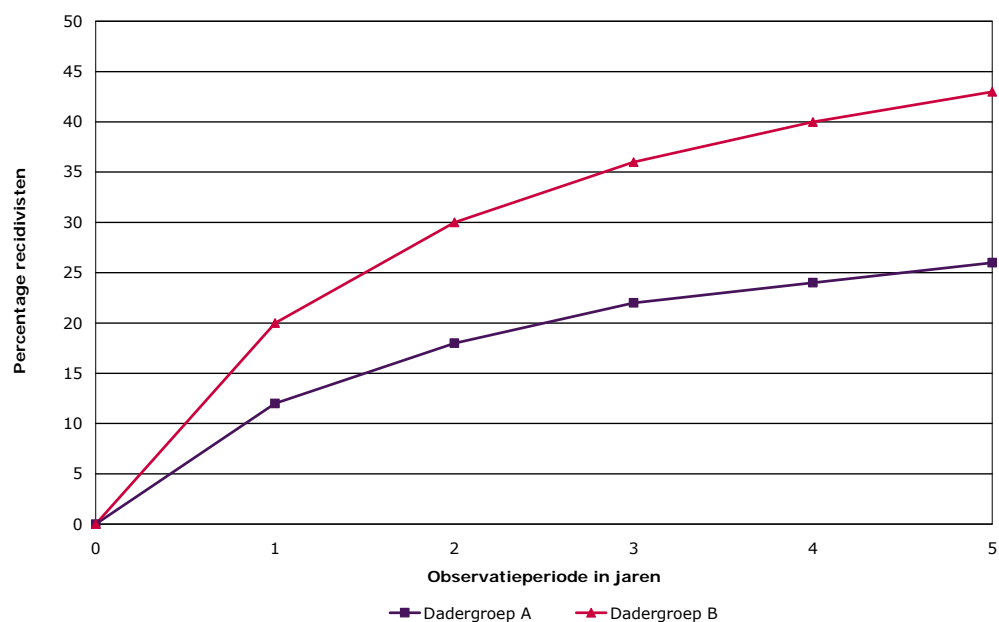
Figuur 1 Prevalentie van algemene recidive onder dadergroep A en B (fictieve cijfers)
